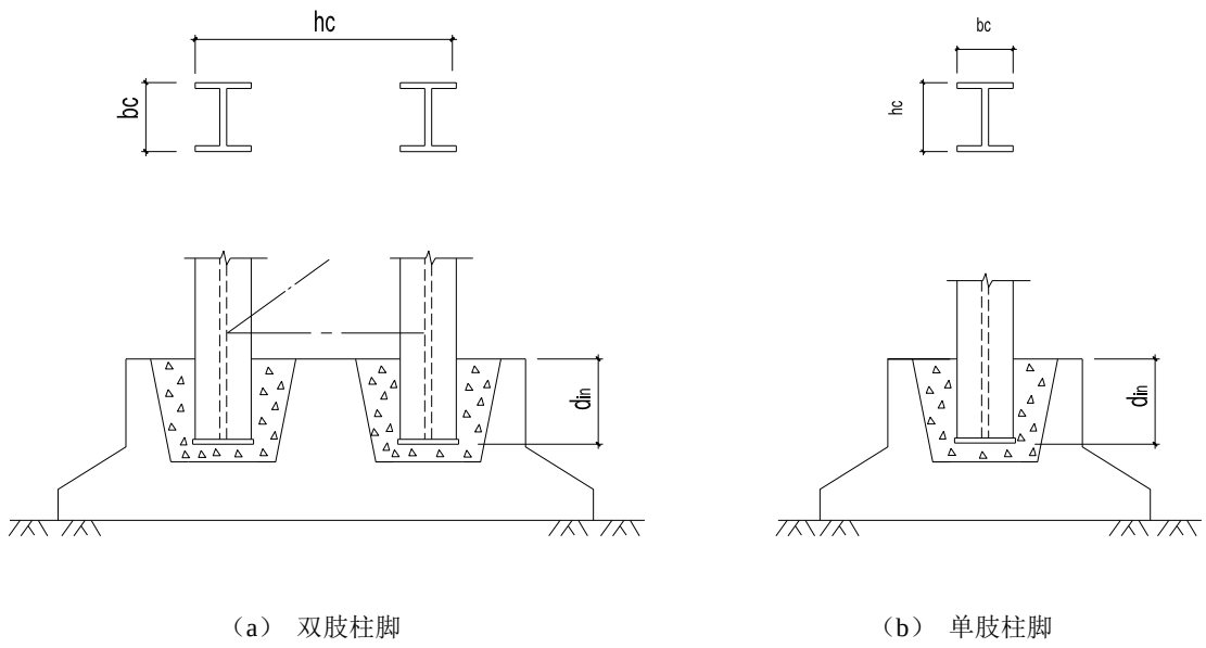
图 26 插入式柱脚
