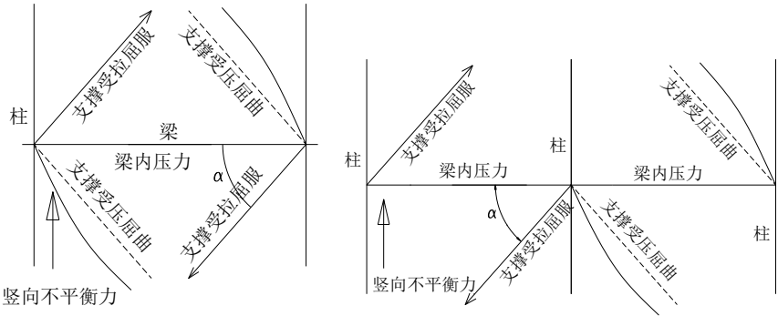
图 48 交叉支撑节点不平衡力示意
