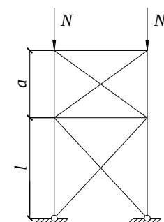
图 8 有支撑的二段柱
