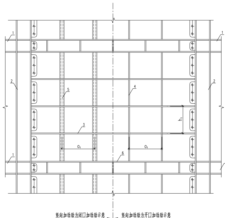
图 10 加劲钢板剪力墙示意
