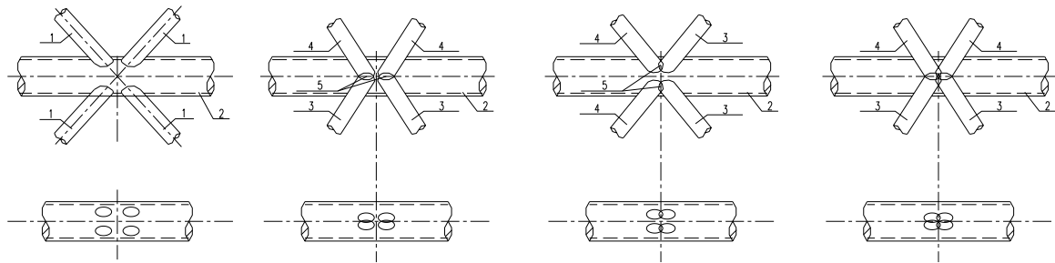
(a) 空间 KK-Gap 形节点 (b) 空间 KK-OPOv 形节点 (c) 空间 KK-IPOv 形节点 (d) 空间 KK-Ov 形节点
