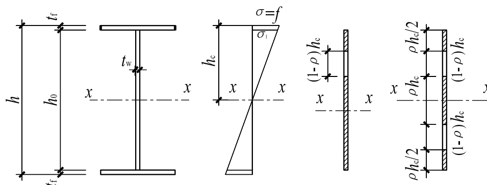
图5 梁截面模量折减系数简化计算简图
