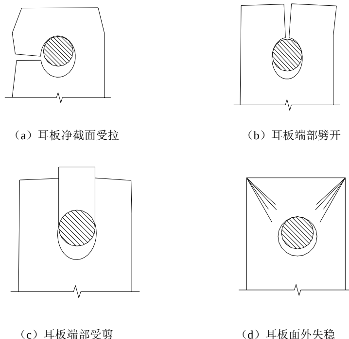
图 16 销轴连接中耳板四种承载力极限状
