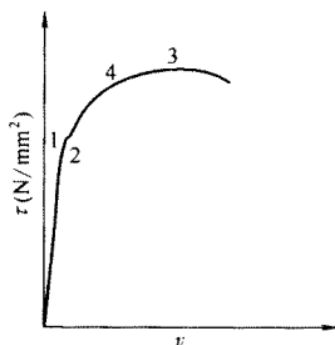
图 15 单个螺栓受剪时的工作曲线
