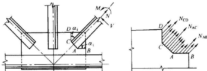
图 17 节点板受拉计算简图
