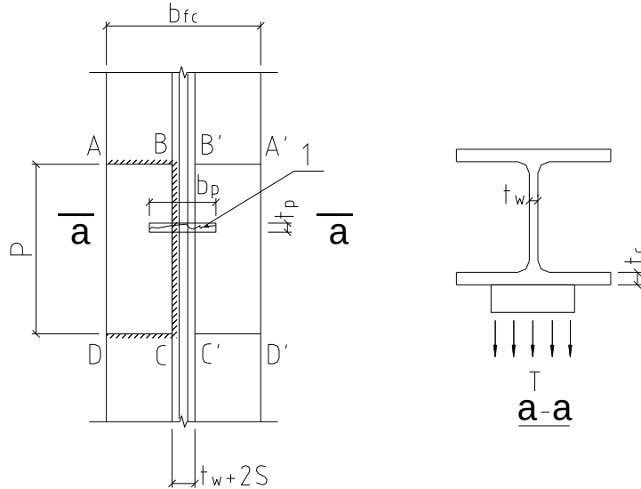
图 18 柱翼缘受力示意
