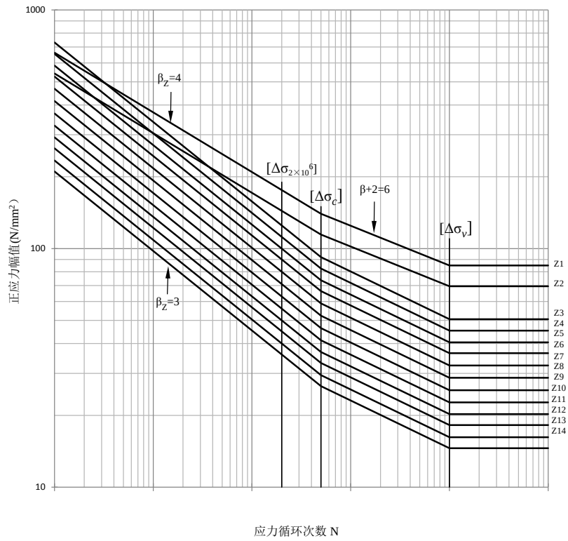
图 45 关于正应力幅的疲劳强度 S-N 曲线
