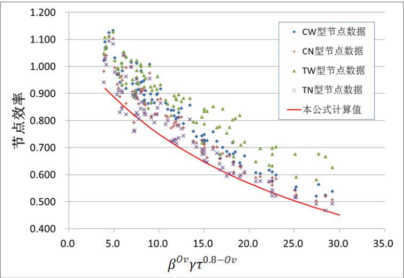
图 36 本标准公式计算值与四种类型搭接节点有限元数据的对比
