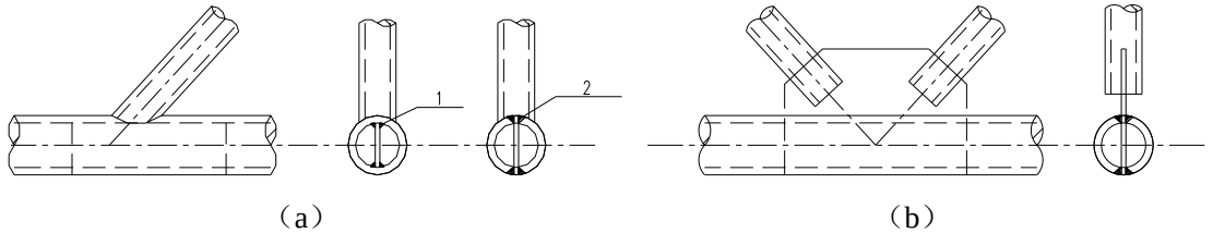
图 34 主管内纵向加劲的节点 1-内部焊接; 2-开槽后焊接
