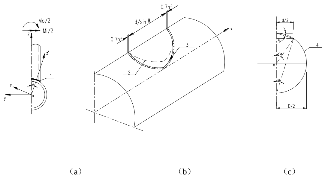
图 42 焊缝截面的简化
