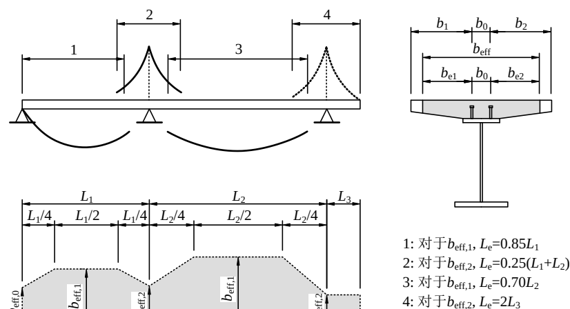
图 43 混凝土翼板的等效跨径及有效宽度（欧洲组合结构设计规范 EC4）
