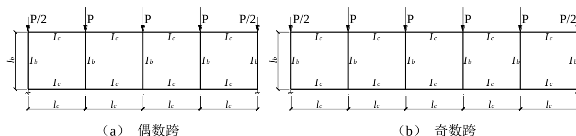
图 51 多跨空腹桁架
