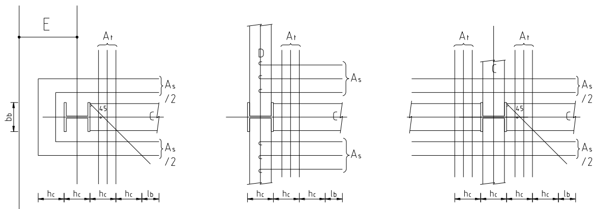
图 49 钢柱周边钢筋锚固示意图
