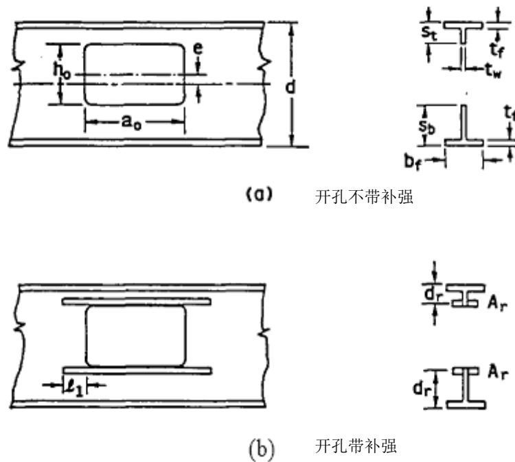
图6 腹板开孔梁计算几何图形
