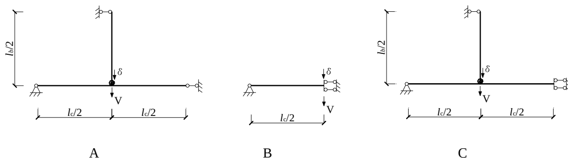
图 53 子结构模型
