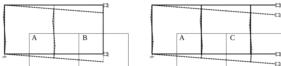
图 52 空腹格构梁的变形模式
