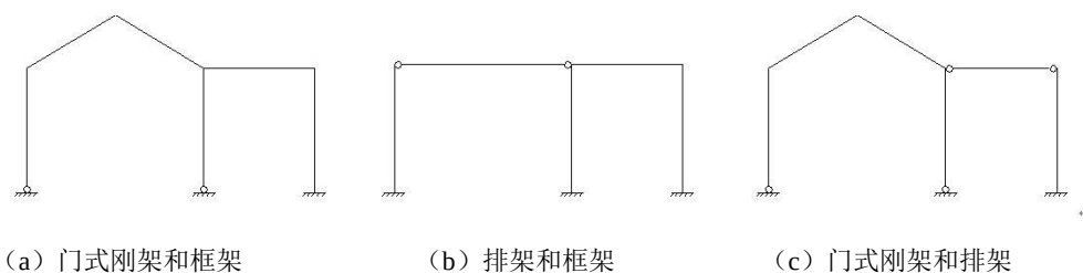
图 50 混合形式
