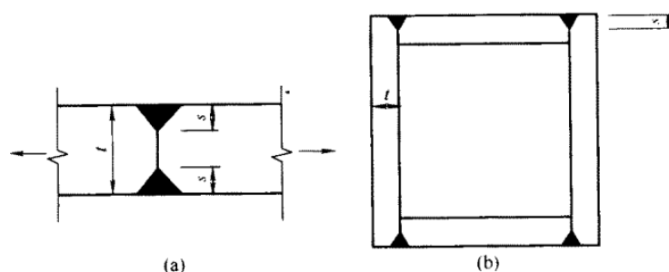
图 14 部分焊透的对接焊
