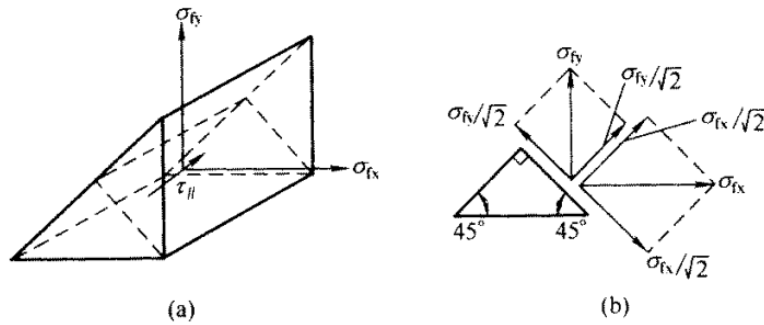
图 12 角焊缝 \sigma_{fx} 、 \sigma_{fy} 、 \tau_f 共同作用
