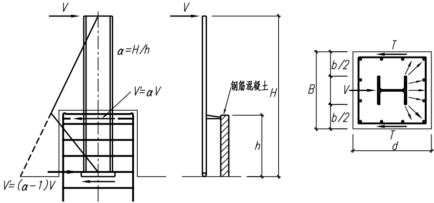
图 23 外包式柱脚的计算概念图
