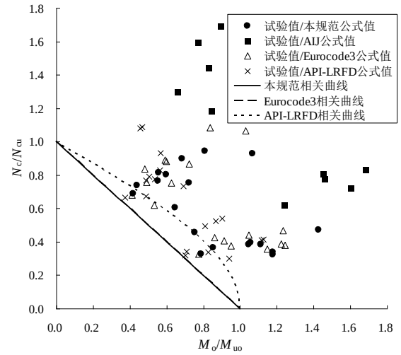
图 39 N_c - M_o 相关方程与试验数据的比较
