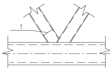
图 33 隐蔽部分施焊时搭接支管断开示意
