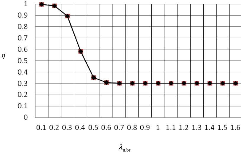
图 47 受压支撑卸载系数与支撑正则化长细比的关系
