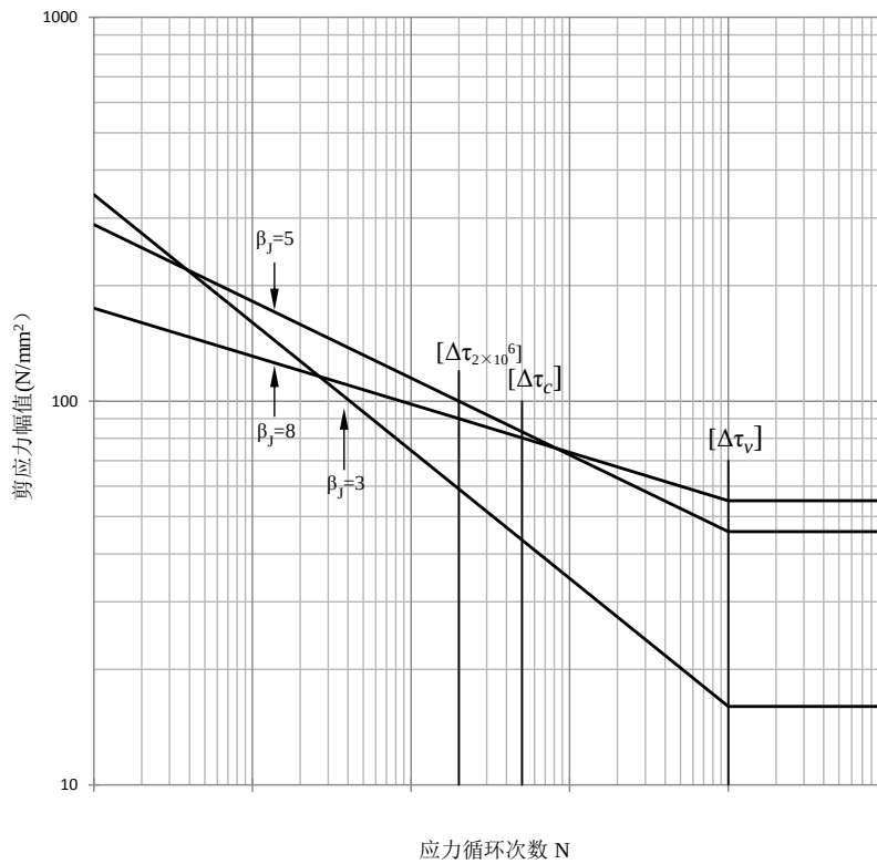
图 46 关于剪应力幅的疲劳强度 S-N 曲线
