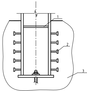
图 25 埋入式柱脚
