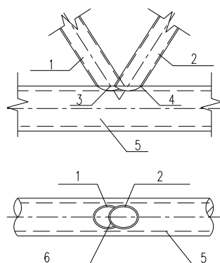
图 31 搭接连接的隐蔽部位
