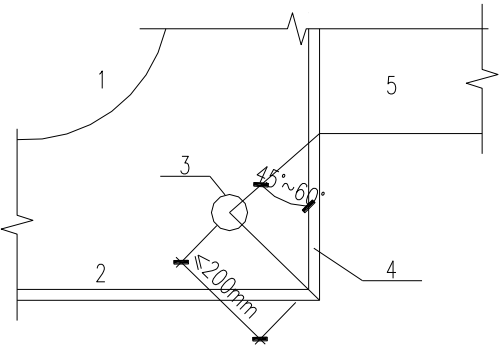
图 44 矩形钢管混凝土柱隔板开孔
