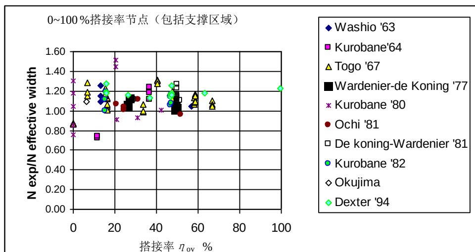
图 30 搭接率对节点承载力的影响
