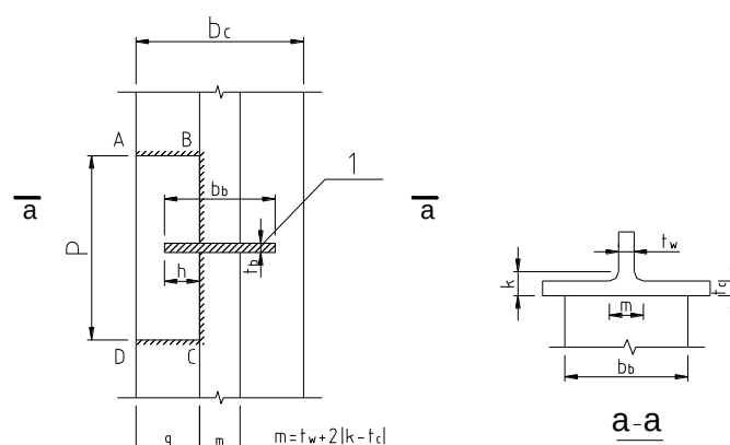
图 19 柱翼缘在拉力下的受力情况
