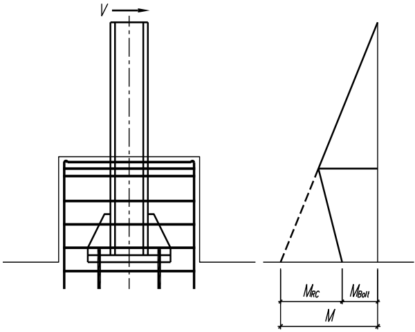
图 24 外包式柱脚地脚螺栓的计算方法
